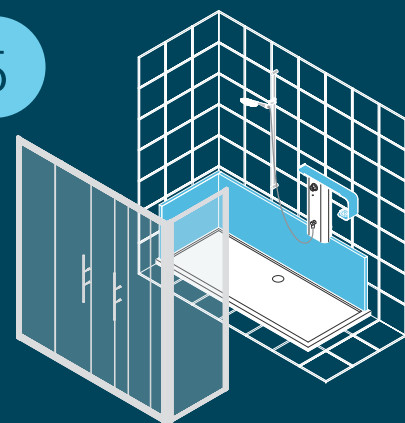
5. ASSEMBLAGGIO ED INSTALLAZIONE BOX DOCCIA 5. SHOWER SYSTEM INSTALLATION
