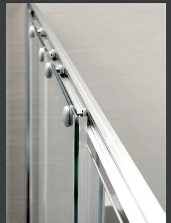
Sistema di scorrimento ad alta durata su cuscinetti a sfere in inox, con regolazione su eccentrico.
