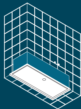
2. ADEGUAMENTO SCARICO A PAVIMENTO E POSA PIATTO DOCCIA 2. DRAIN AND SHOWER TRAY INSTALLATION
