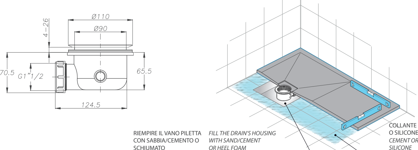
SCHEDA TECNICA PILETTA DRAIN TECHNICAL DATA SHEET
