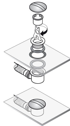
PARTICOLARE PILETTA PARTICULAR DRAIN
