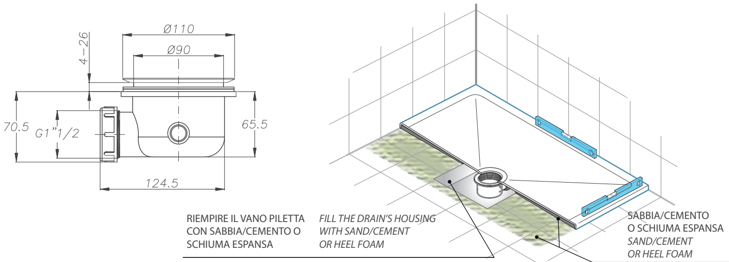
SCHEDA TECNICA PILETTA DRAIN TECHNICAL DATA SHEET
