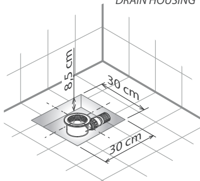
PREDISPOSIZIONE INCASSO PILETTA DRAIN HOUSING
