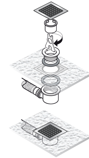
PARTICOLARE PILETTA PARTICULAR DRAIN
