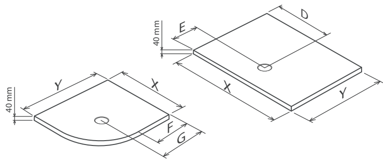
PARTICOLARE PILETTA PARTICULAR DRAIN
