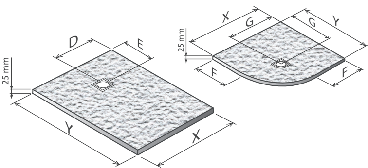
PREDISPOSIZIONE INCASSO PILETTA DRAIN HOUSING
